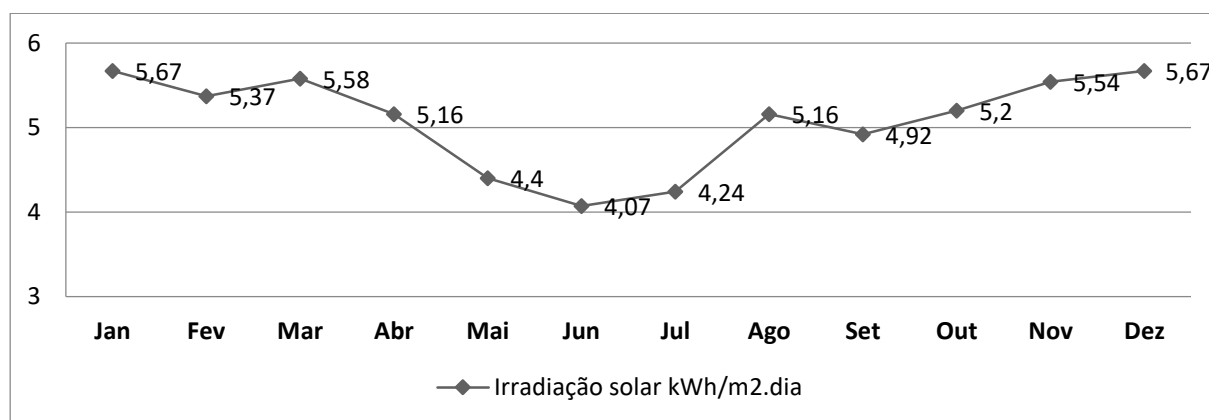
Figura 4. Irradiância solar no plano inclinado na latitude de Tupãssi-PR, durante os meses do ano de 2018 - Atlas de Energia Solar do Paraná.
