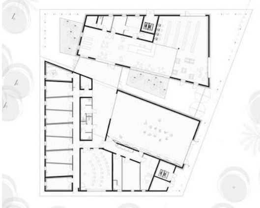
Imagem 06: Planta baixa.
