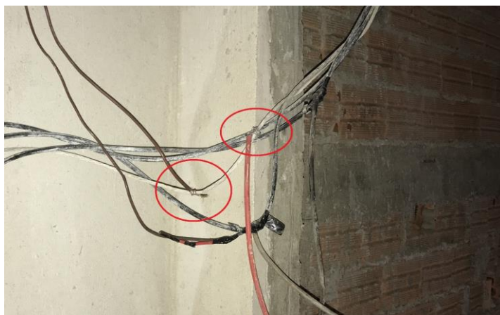
Figura 11 - Amostra C, parte exposta de viação sem isolamento adequado.
