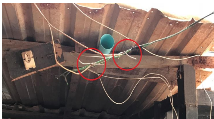
Figura 10 - Amostra A, parte exposta de viação sem isolamento adequado.
