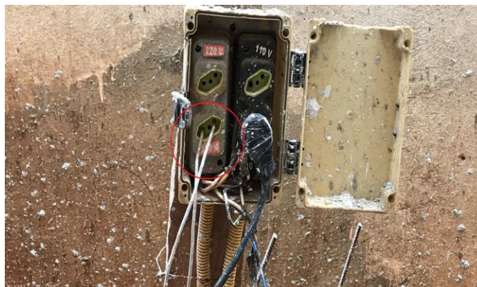
Figura 18 - Amostra A, condutor conectada diretamente em ponto tomada. Fonte: Autor (2018).
