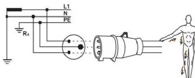
Figura 04 - Proteção contra contatos diretos.
