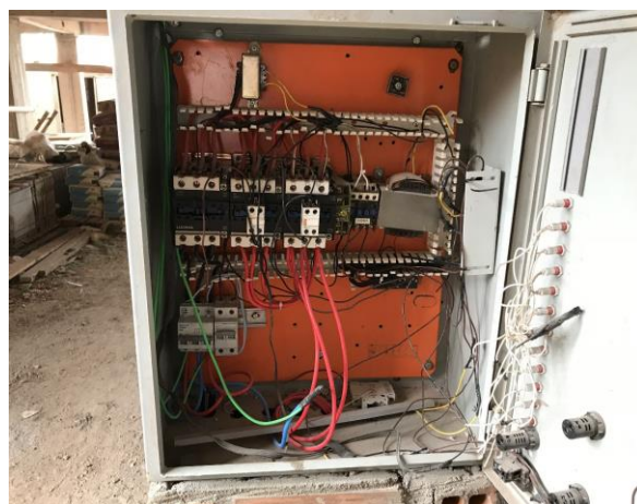
Figura 15 - Amostra B, quadro de distribuição do elevador de carga.
