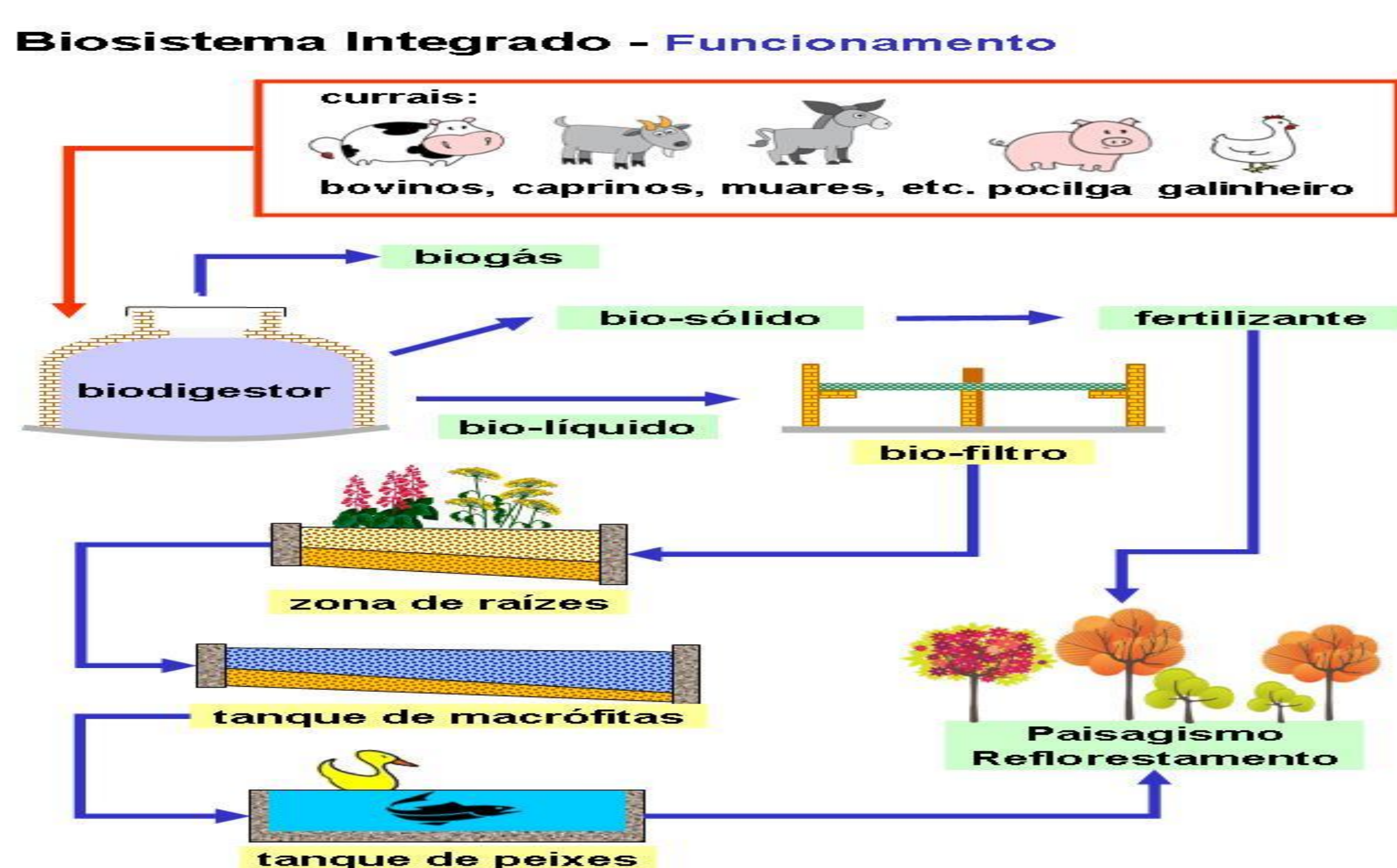
Figura1. Biossistema Integrado - Fluxograma
